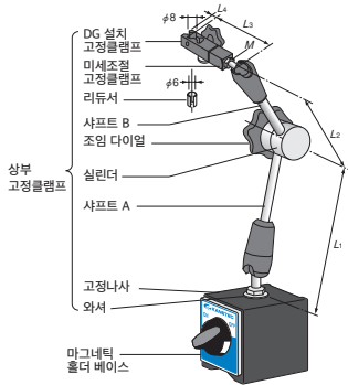
<명칭/치수도>
